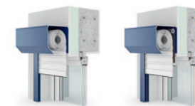
Vorbaukasten 45° 45° abgeschrägt, rollgeformt oder stranggepresst, wahlweise mit integriertem Fliegengitter.
