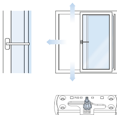
Schiebetür geöffnet
