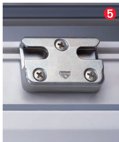
Sicherheitsschließzapfen mit Pilzkopf sorgen in Verbindung mit Sicherheitsschließstücken für hohe Sicherheit
